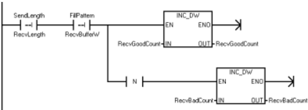
程序段 27: 在所有情况下都进入“空闲”状态。
