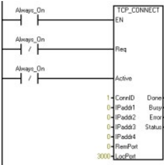
程序段 8：如果 Done 为 TRUE，则表示 CPU 已建立该连接，所以继续进入“空闲”状态。
