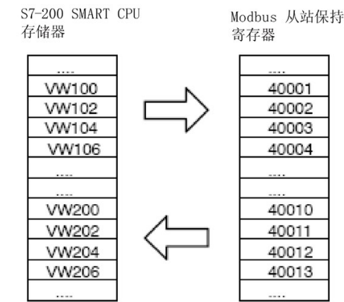
图 9-1 程序数据传送示例
