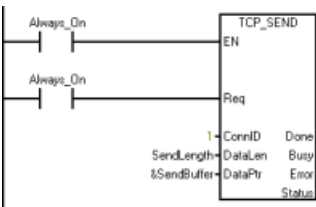
程序段 16: 如果 Done 为 TRUE，则发送操作已完成（几乎不会很快完成），之后进入下一次扫描的“接收”状态。
