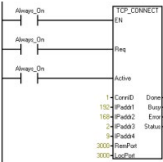
程序段 5： 如果 Done 为 TRUE，则 CPU 建立该连接以进入“空闲”状态。 如果 Busy 为 TRUE，则 CPU 进入“连接等待”状态以等待连接的建立。 如果 Error 为 TRUE，则可能输入参数有误，检查输入参数以决定 CPU 接下来要进入哪个状态。
