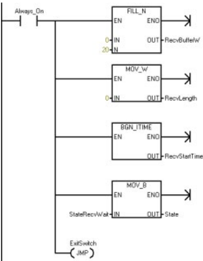
程序段 22： 状态“接收等待”... 停留在该状态直到接收到某些数据或超时。
