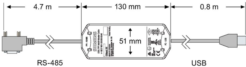
图 A-1 USB/PPI 多主站电缆尺寸和 LED
