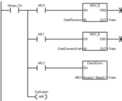
程序段 6：状态“连接等待”...
