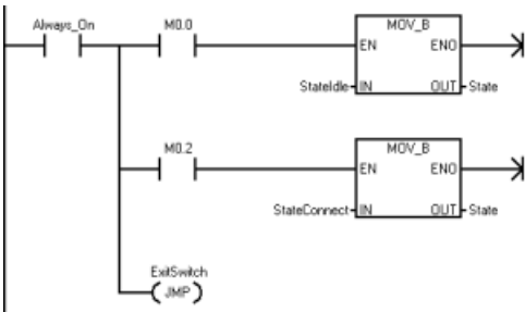
程序段 9：状态“空闲”...
