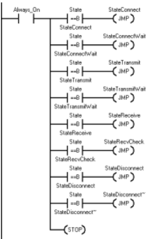
程序段 3: 状态连接...
