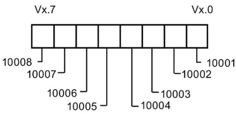
压缩字节的格式（离散量输入地址）
