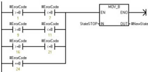
程序段 4：如果连接出现问题，则程序会返回错误 15 和 31。断开并重新连接以纠正这个问题。
