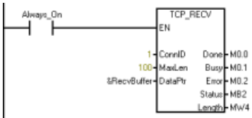
程序段 11：如果 Done 为 TRUE，则表示 CPU 已接收到新数据，之后进入“接收检查”状态。
