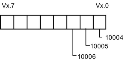
压缩字节的格式（从地址 10004 开始的离散量输入）
