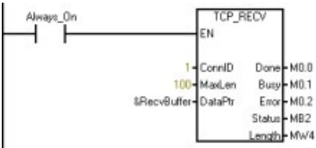
程序段 24： 如果 Done 为 TRUE，则该指令已接收到新数据，之后进入“接收检查”状态。 如果 Busy 为 TRUE，则停留在“接收”状态，直到停留时间达到接收超时值。如果停留在该状态的时间已超时，则断开与设备的连接，之后再重新与其建立连接。 如果 Error 为 TRUE，则检查错误代码以确定接下来的操作。
