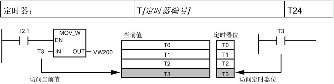
图 4-2 访问定时器位或定时器的当前值
