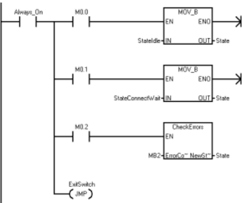
程序段 6: 状态“连接等待”...
