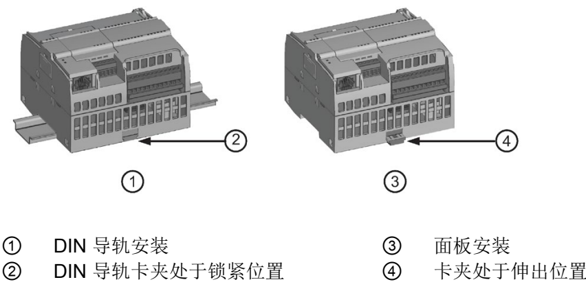
图 3-1 在 DIN 导轨或面板上安装
