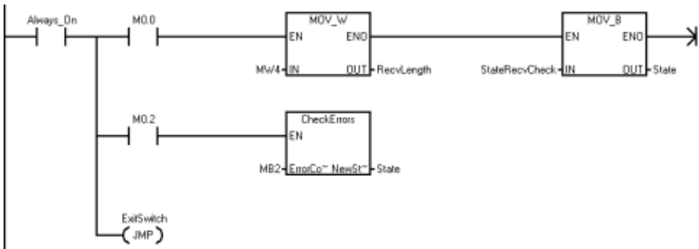
程序段 12：状态“接收检查”...
