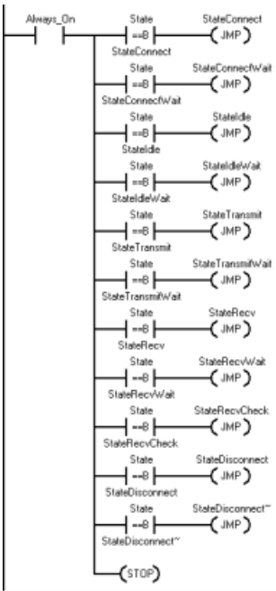
程序段 3： 状态“连接”... 启动连接过程。
